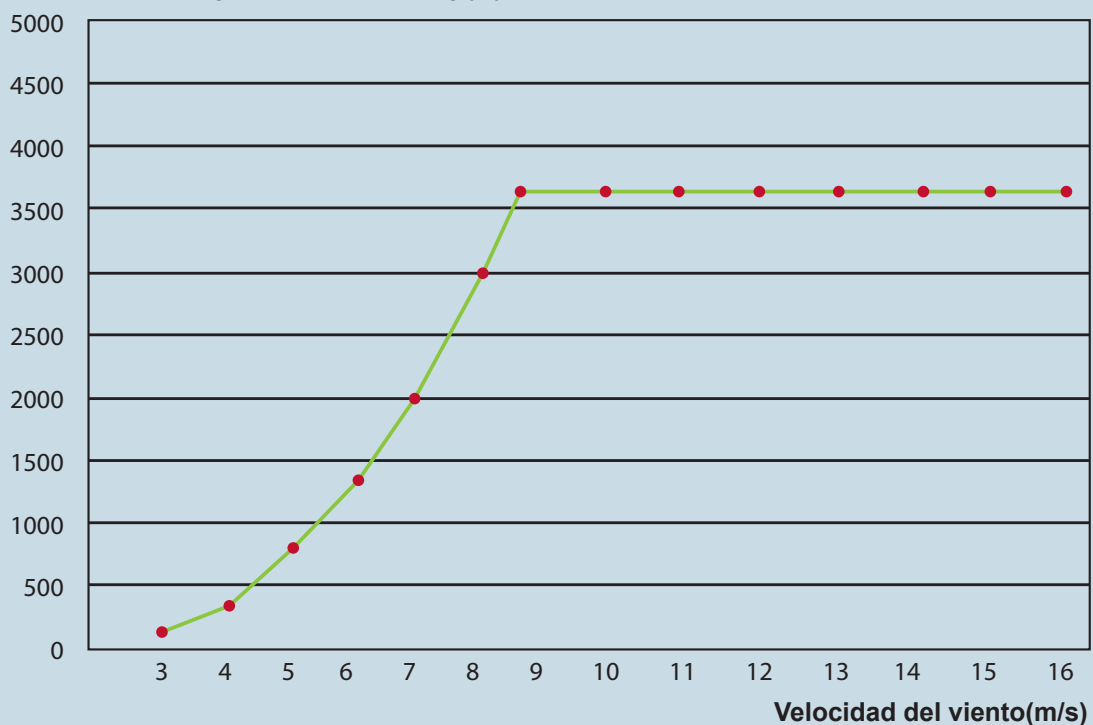
Curva de potencia de salida p(w)
